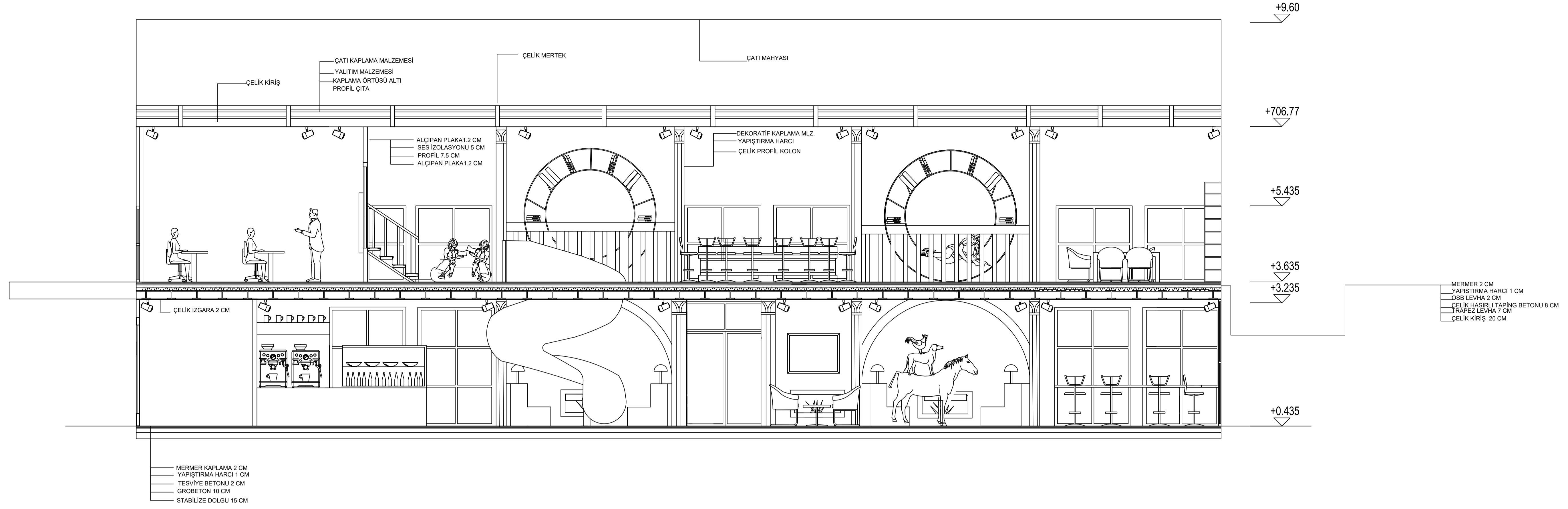
AA KESİTİ
