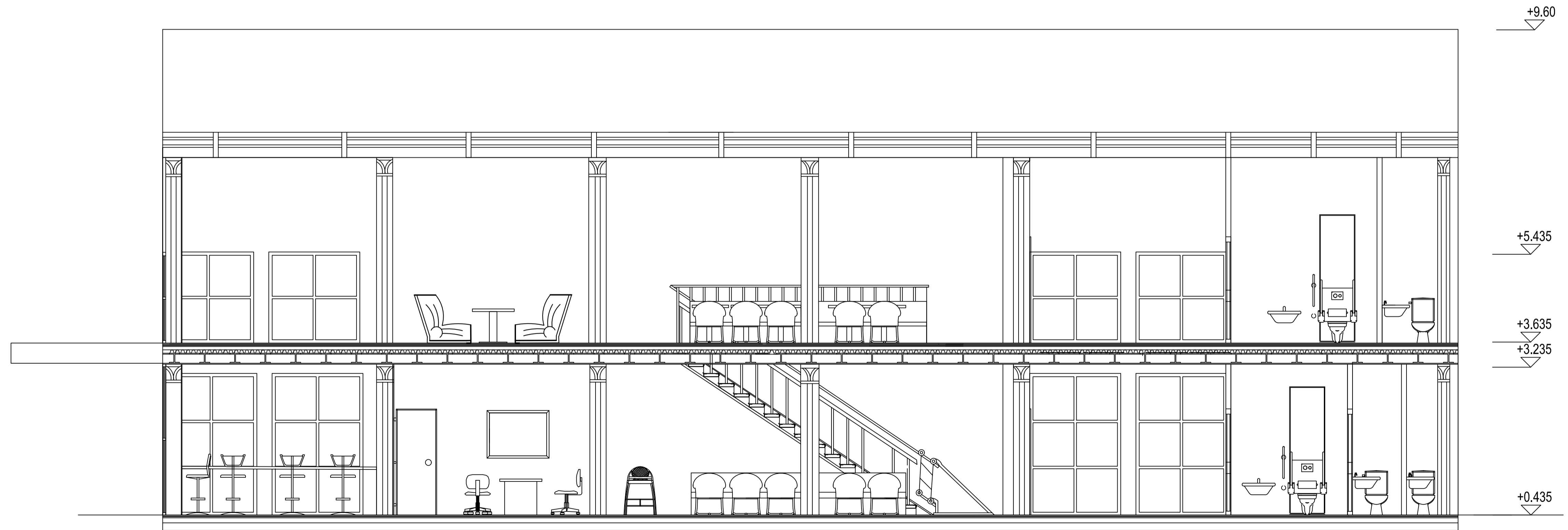
AA KESİTİ
